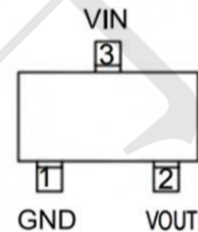
SOT23-3L & SOT23
